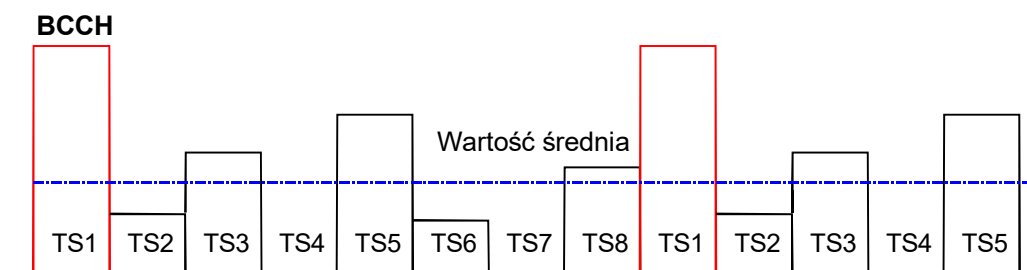
Rys. 1: Podział czasowy transmisji nadajnika stacji bazowej GSM
